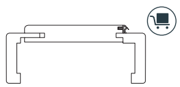
Futter Rundform (RF), Bekleidungsbreite 60 mm
