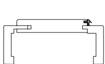
Futter kleine Rundkante (KR), Bekleidungsbreite 60 mm
