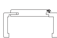
Futter Rundform (RF), Bekleidungsbreite 80 mm
