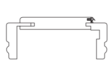
Futter Profiliert (PR), Bekleidungsbreite 65 mm
