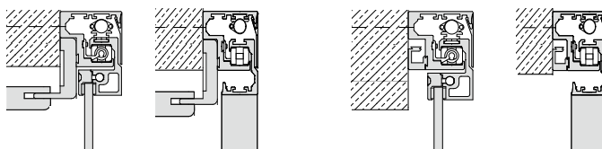
Montage mit DUFU
