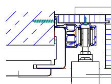
Montage mit Schiebetürfutter für Holztür
