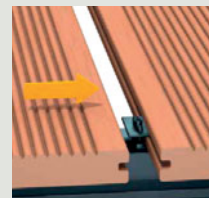
einschieben...
